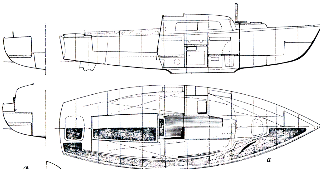
327a Victoire 22, ontwerp D. Koopmans. L.o.a. 6.60 m, l.w.l. 5.60 m, b. 2.20 m, d. 0.95 m, w.v. 0.95 t, ba. 400 kg, schaal 1 : 60; b z.o. 19.50 m 2 , gr.z. 9.75 m 2 , f. 6.60 m 2 , gen. 9.75 m 2 , schaal 1 : 120
