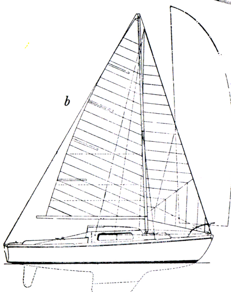
327a Victoire 22, ontwerp D. Koopmans. L.o.a. 6.60 m, l.w.l. 5.60 m, b. 2.20 m, d. 0.95 m, w.v. 0.95 t, ba. 400 kg, schaal 1 : 60; b z.o. 19.50 m 2 , gr.z. 9.75 m 2 , f. 6.60 m 2 , gen. 9.75 m 2 , schaal 1 : 120
